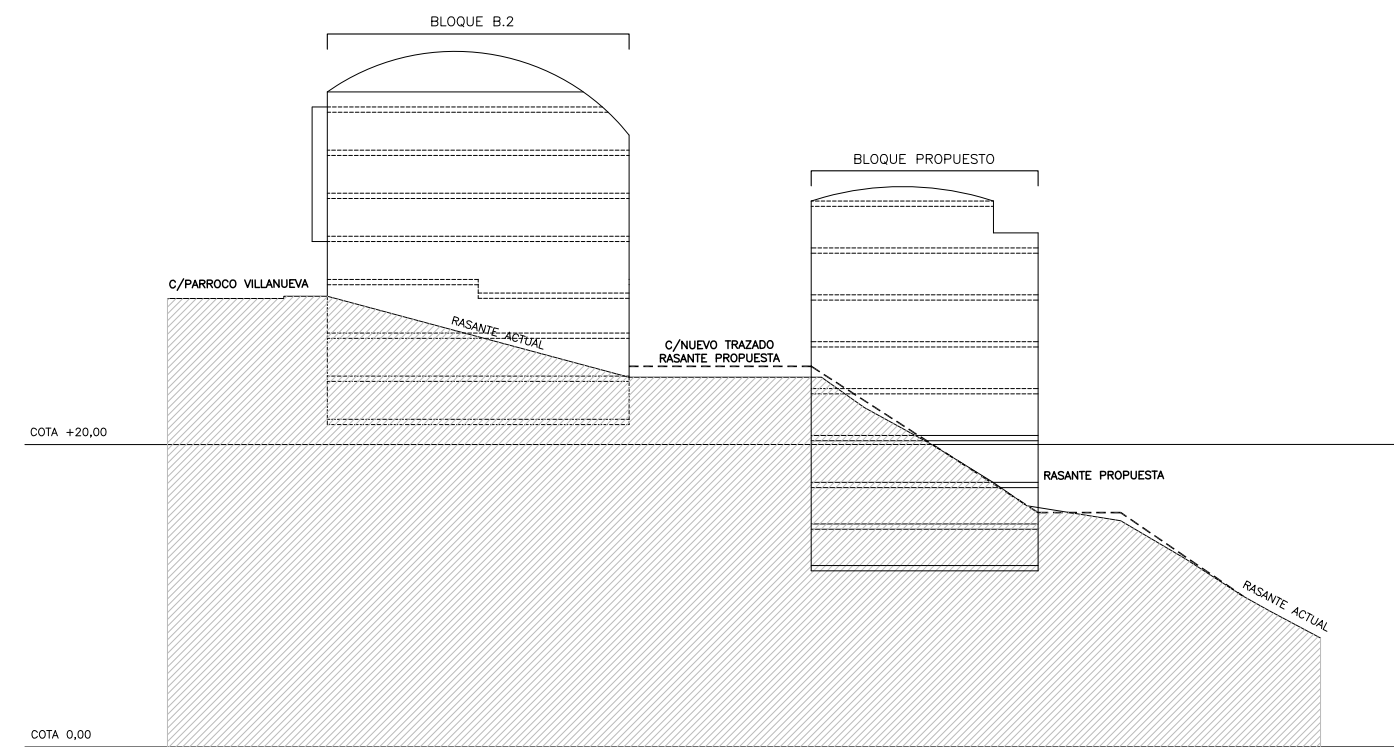
SECCIÓN T.3
