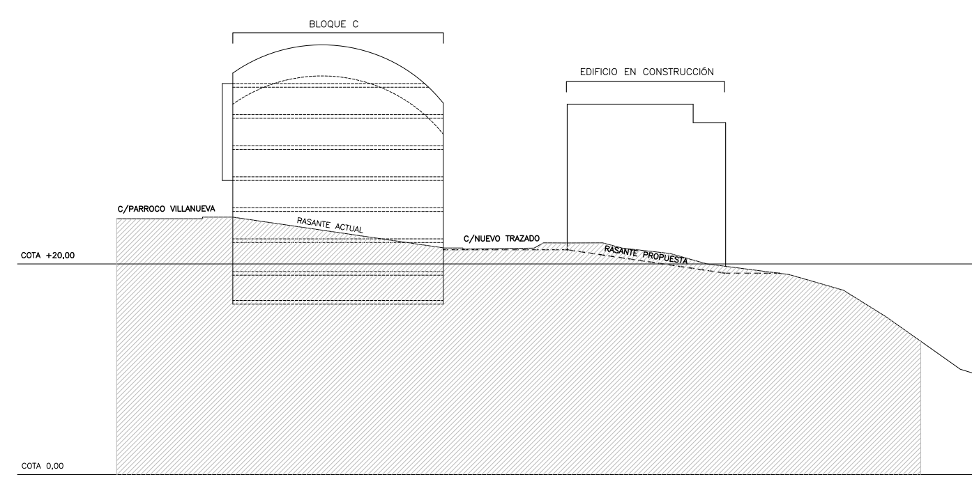
SECCIÓN T.5
