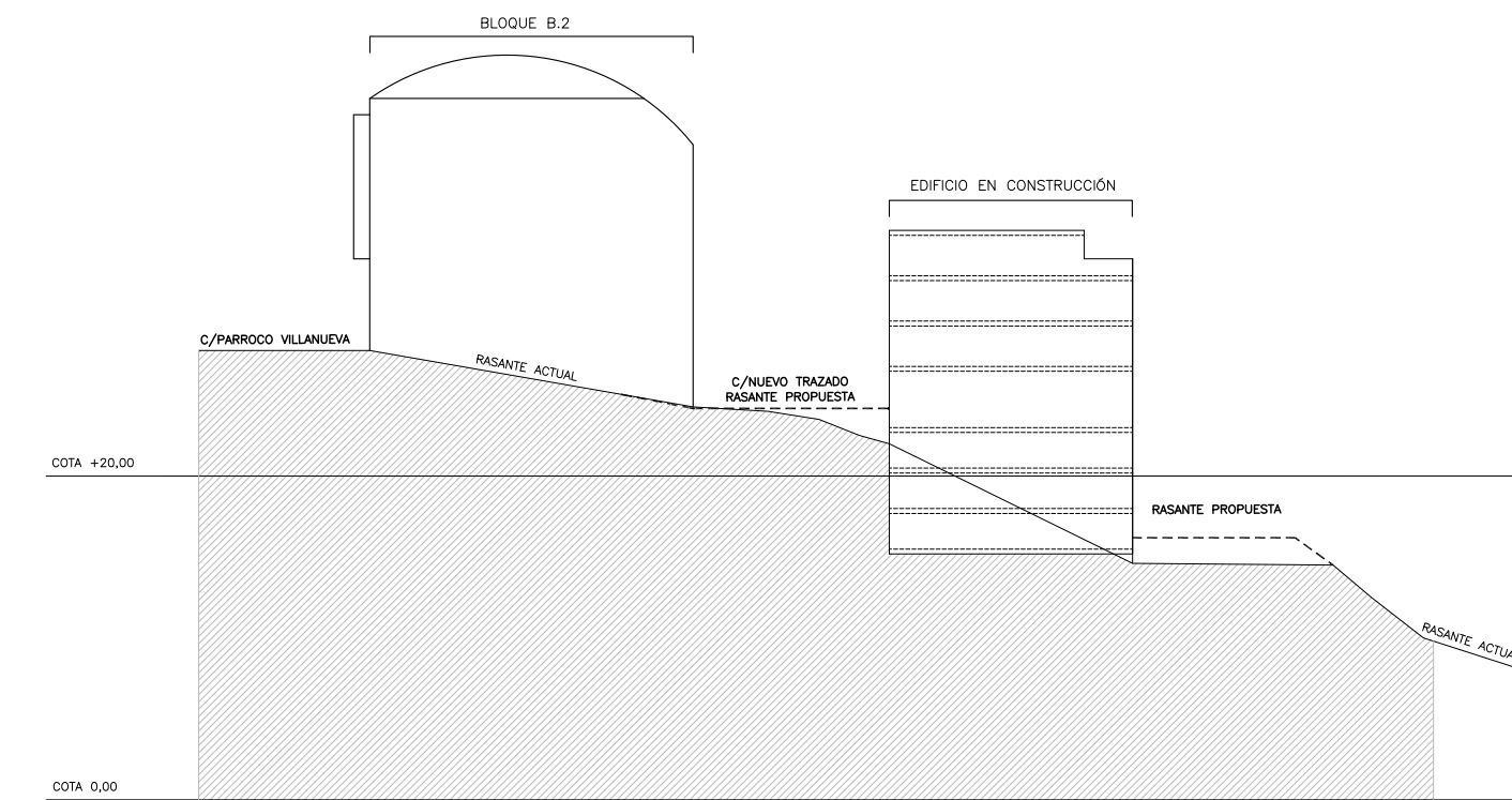
SECCIÓN T.4
