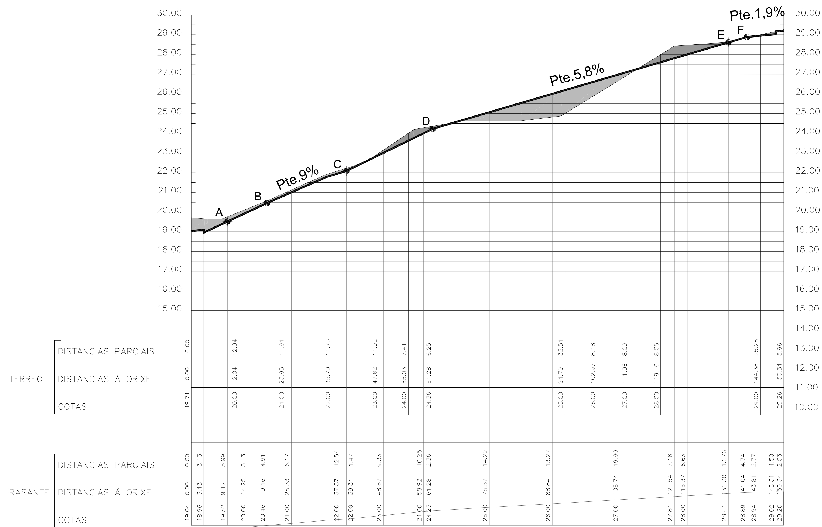
PERFIL LONXITUDINAL RUA NOVO TRAZADO
