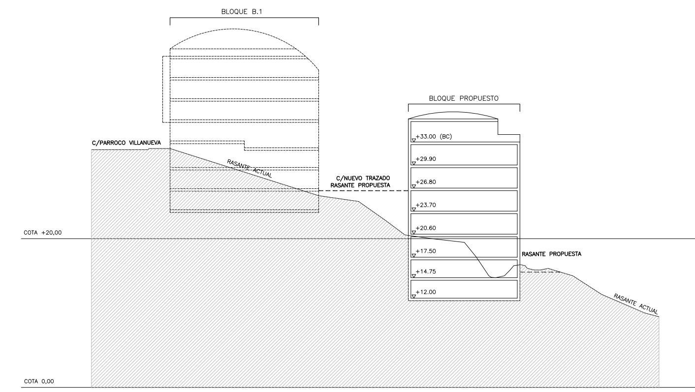
SECCIÓN T.2
